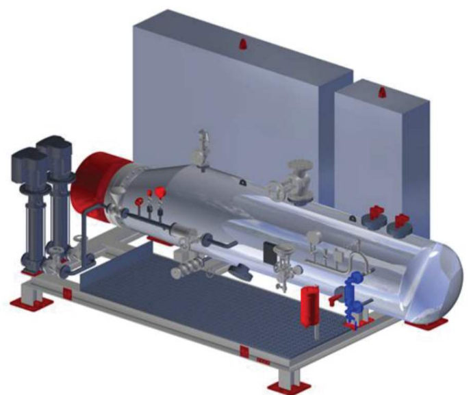
Caldeiras Electricas
